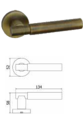
Maniglia su rosetta Handle on roses
