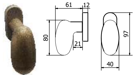
Maniglia per finestra Window handle
