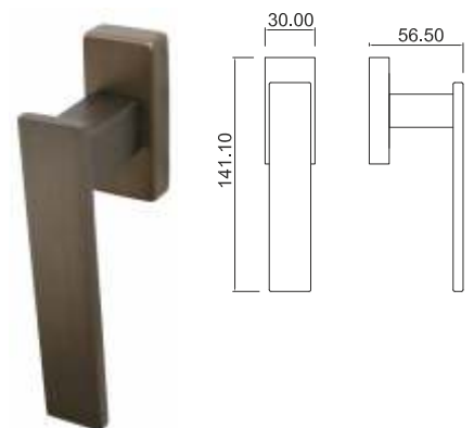
Maniglia per finestra Window handle
