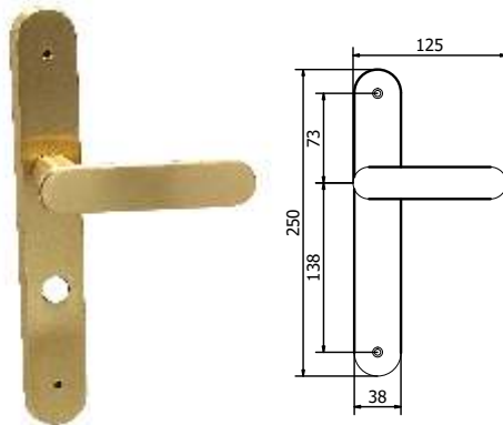
Maniglia su placca Handle on plate
