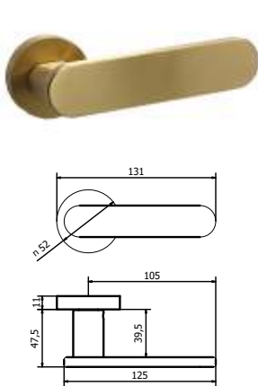
Maniglia su rosetta Handle on roses
